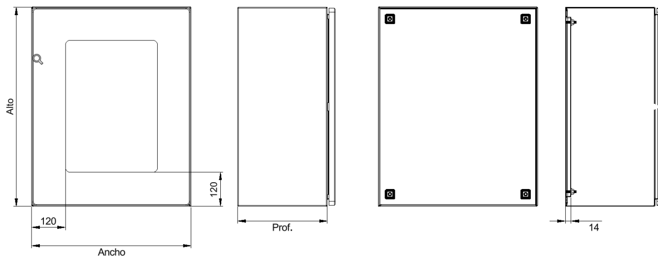
Figura 1: gabinetes de altura menor a 900 mm 4 tornillos de fijación
